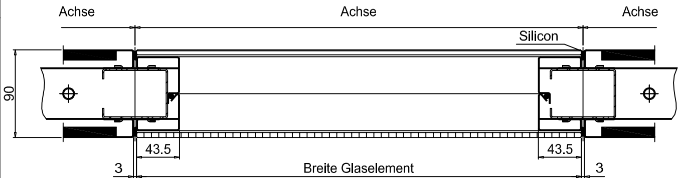
Schnitt A-A
